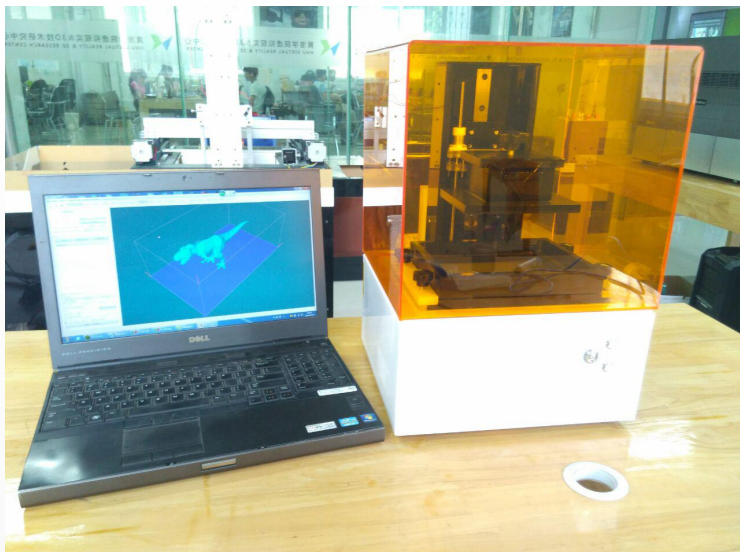
桌面级DLP光固化3D打印机
